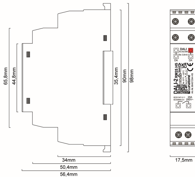
dimensions RM25 HS
