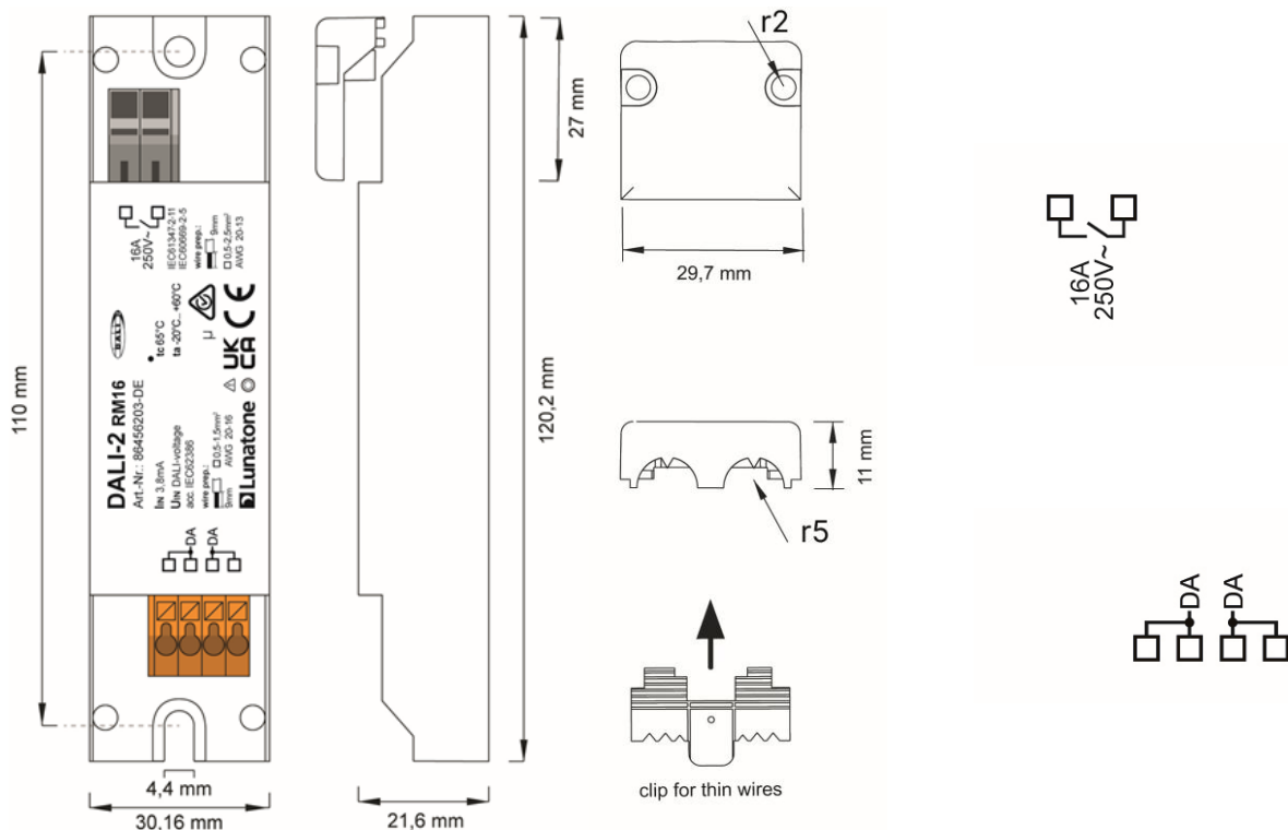
dimensions RM16 DE
